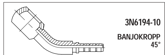
Artikel nr Beteckning 3N6194-10-03 BANJO 10MM 45° 1/8" 3N6194-10-04 BANJO 10MM 45° 3/16"
