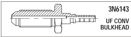
Artikel nr Beteckning 3N6143-31-03 M10x1 UF CONV BULKHEAD 1/8"
