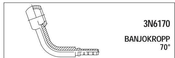
Artikel nr Beteckning 3N6170-10-03 BANJO 10MM 70° 1/8" 3N6170-10-04 BANJO 10MM 70° 3/16"
