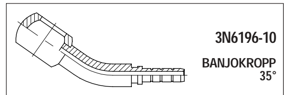
Artikel nr Beteckning 3N6196-10-03 BANJO 10MM 35° 1/8"
