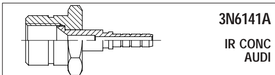
Artikel nr Beteckning 3N6141-31-03A M10x1 IR CONC AUDI 1/8"
