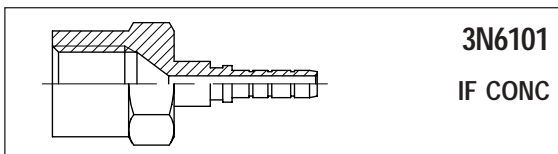
Artikel nr Beteckning 3N6101-31-03 M10x1 IF CONC 1/8"
