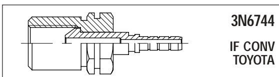
Artikel nr Beteckning 3N6744-31-03 M10x1 IF CONV TOYOTA 1/8"
