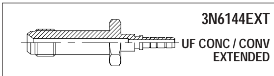
Artikel nr Beteckning 3N6144-31-03EXT M10x1 UF CONV BULKHEAD 1/8"
