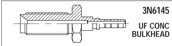
Artikel nr Beteckning 3N6145-31-03 M10x1 UF CONC BULKHEAD 1/8"
